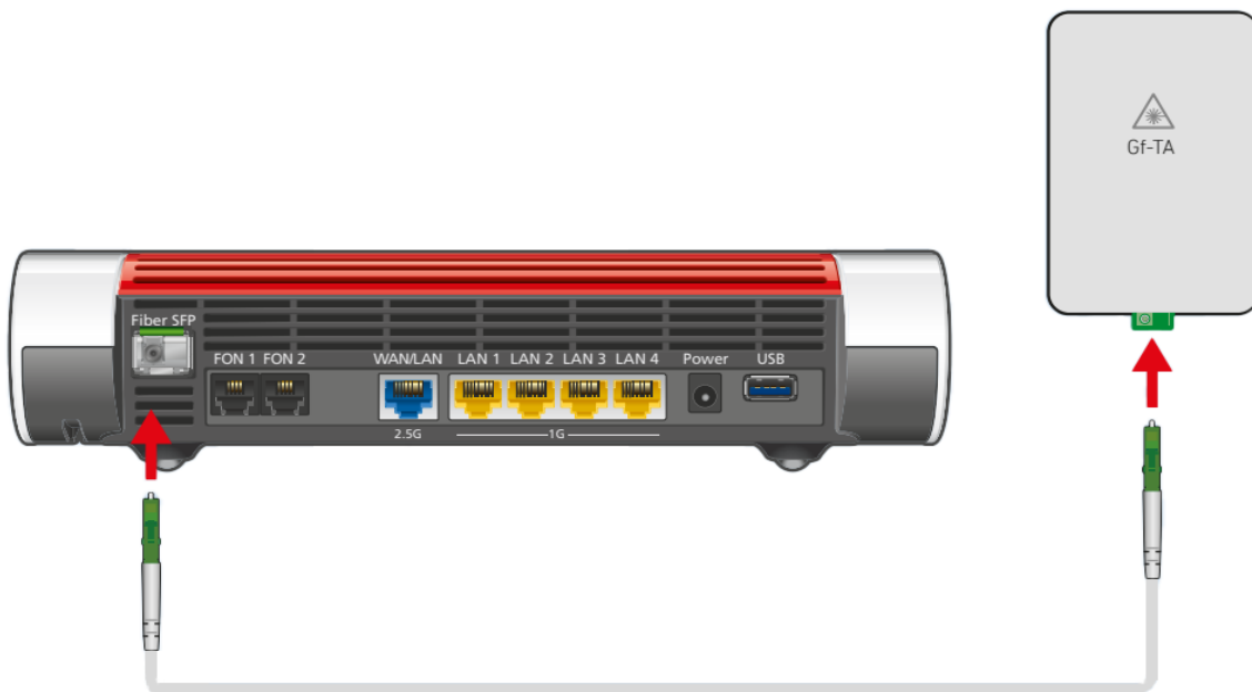
FRITZ!Box mit Glasfaseranschluss verbinden
